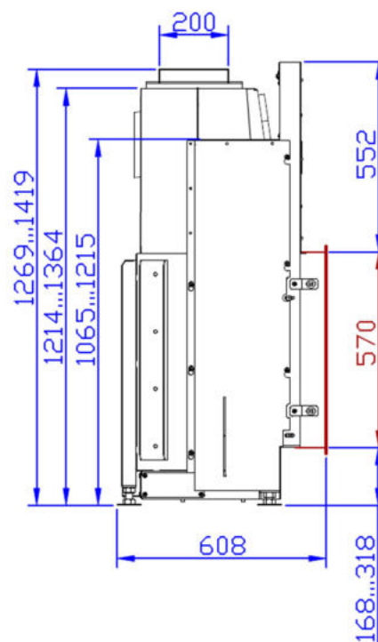
A-A
