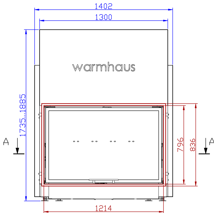
Изображение фронтальное
