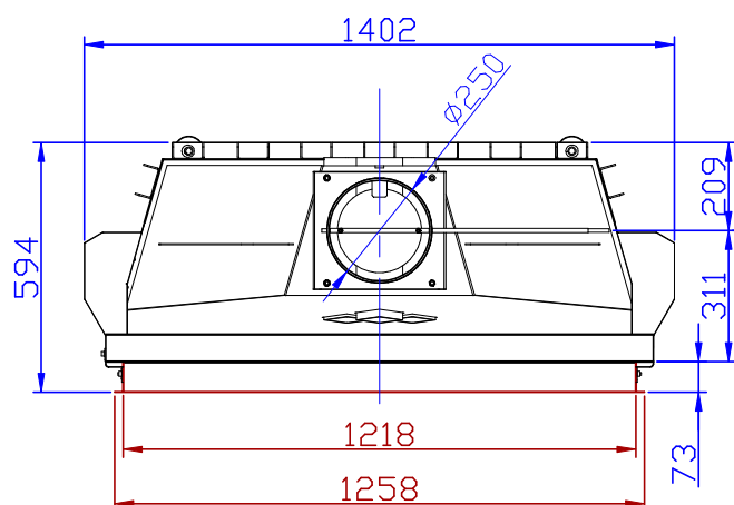
Изображение сверху
