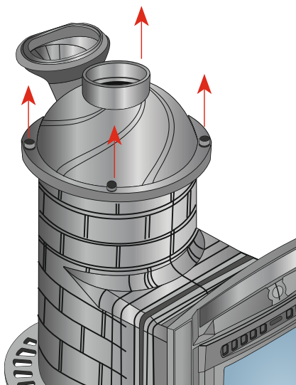
а) Откручиваем 4 болта крепления купола.
