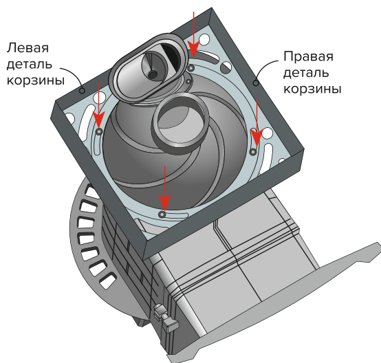
б) Устанавливаем корзину для камней и фиксируем ее теми же болтами крепления купола.
