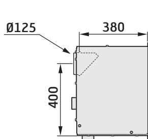
Anslutningsmått
