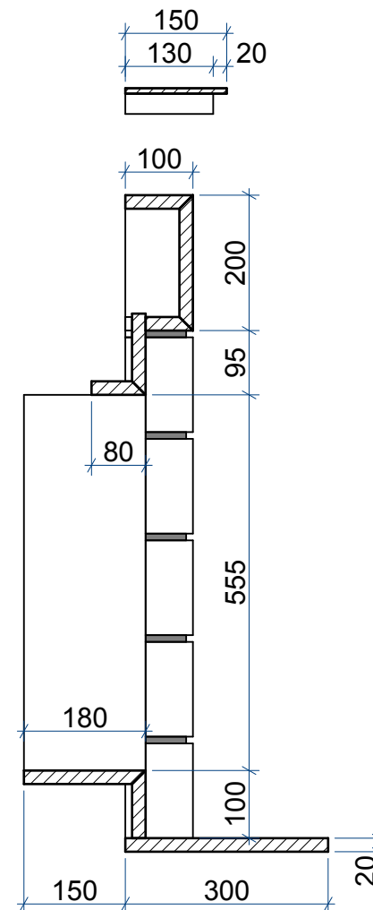
Сечение 2-2
