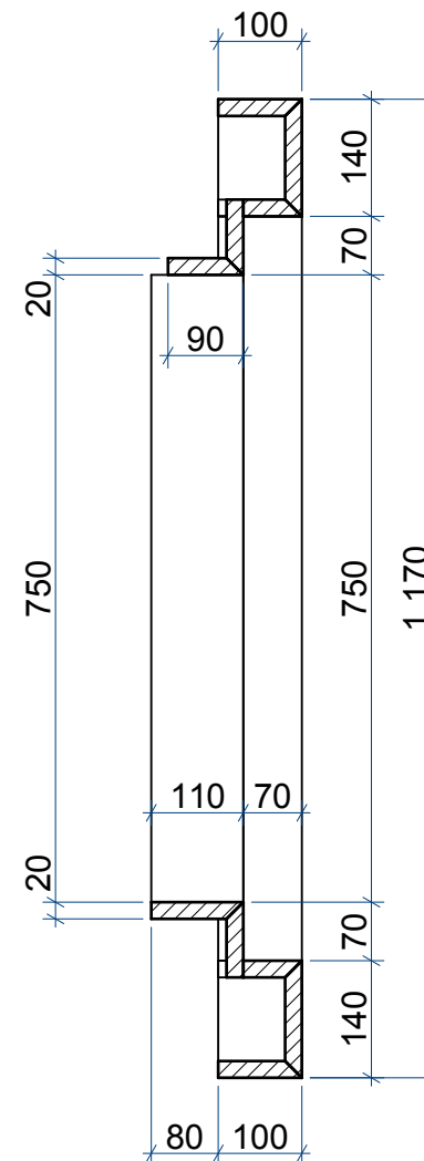
Сечение 2-2
