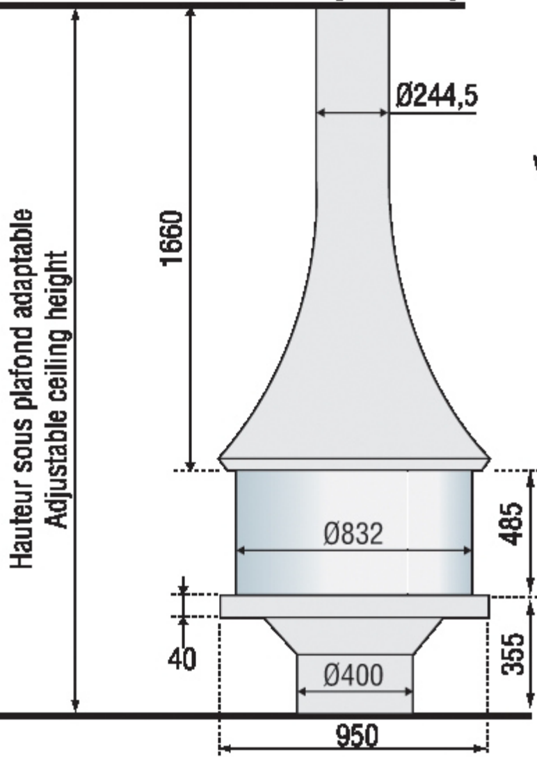
Vue de face [face view]
