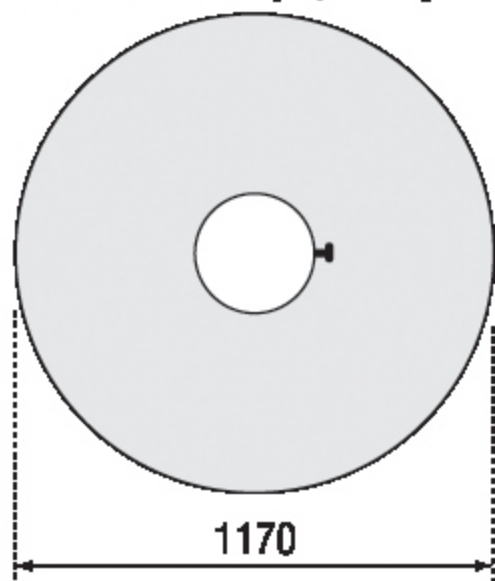
Vue de dessus [top view]
