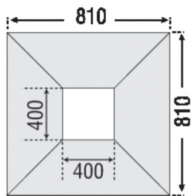
Vue de dessus [top view]
