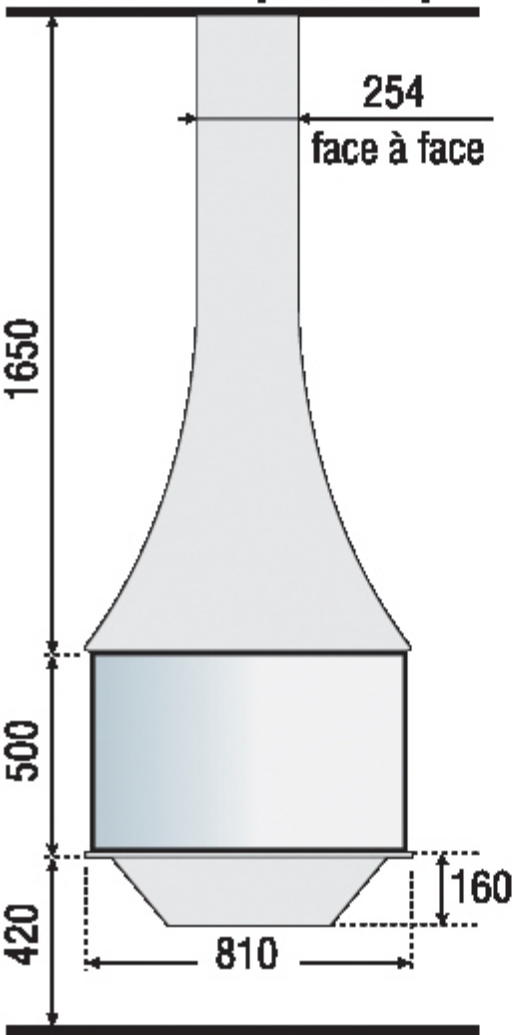
Vue de face [face view]
